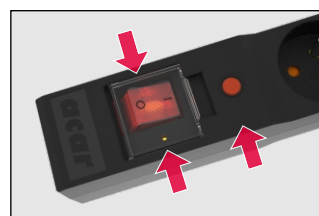
Wzmocniony, dwutorowy, podświetlany wyłącznik sieciowy, zwłoczny bezpiecznik automatyczny, sygnalizacja ochrony przeciwprzepięciowej
